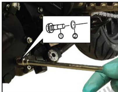
1. Jäähdytysnesteen tyhjennyspultti
